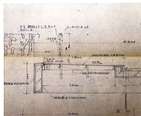
設計図 入口の庇とロ丁文字部分
